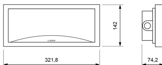
Montaje estanco
